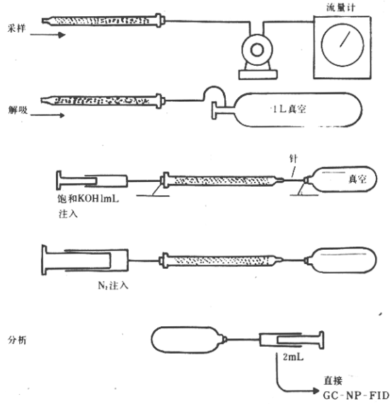
图 2 样品的采集、处理及分析示意图
