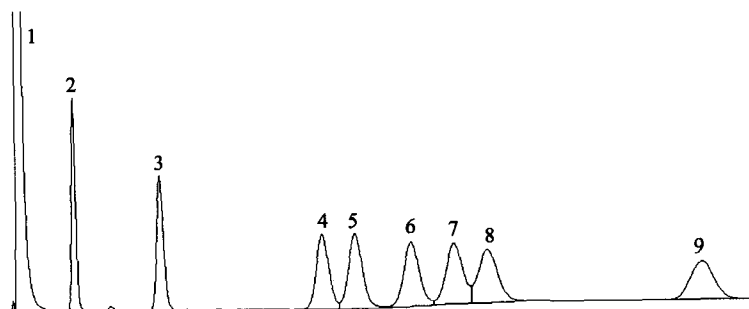
1—二硫化碳；2—苯；3—甲苯；4—乙苯；5—对二甲苯；6—间二甲苯；7—邻二甲苯；8—异丙苯；9—苯乙烯。
