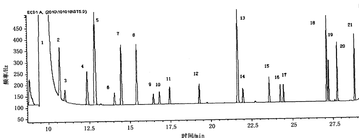
1—二硫化碳（溶剂峰）；2—反式-1,2-二氯乙烯；3—1,1-二氯乙烷；4—顺式-1,2-二氯乙烯；5—三氯甲烷；6—1,2-二氯乙烷；7—1,1,1-三氯乙烷；8—四氯化碳；9—1,2-二氯丙烷；10—三氯乙烯；11—1-溴-2-氯乙烷；12—1,1,2-三氯乙烷；13—四氯乙烯；14—氯苯；15—三溴甲烷；16—1,1,2,2-四氯乙烷；17—1,2,3-三氯丙烷；18—苯基氯；19—1,4-二氯苯；20—1,2-二氯苯+1,3-二氯苯；21—六氯乙烷
